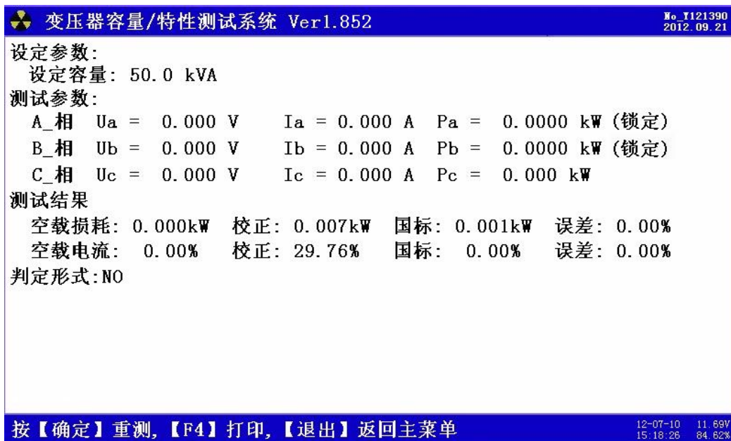
图 16、单相空载—测量结果
