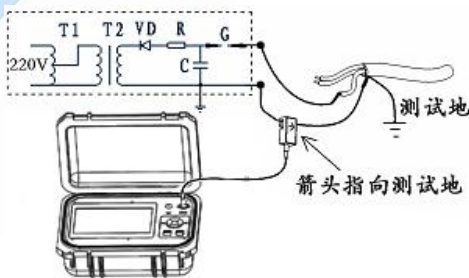
图 4-3-2
