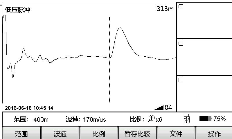
图 2-3-3
