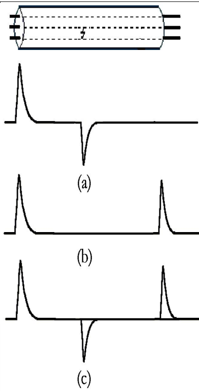
图 5-2-1 二次脉冲法原理示意
