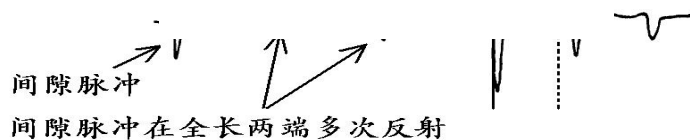
图 4-3-3 典型的直闪法波形：
