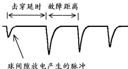
图 4-2-4 冲闪法波形
