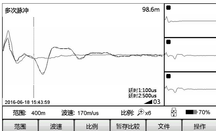
图 5-3-1
