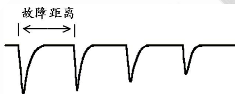
图 4-2-2 直闪法波形
