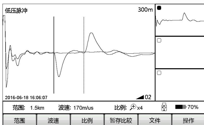
图 3-3-4 相对距离测量
