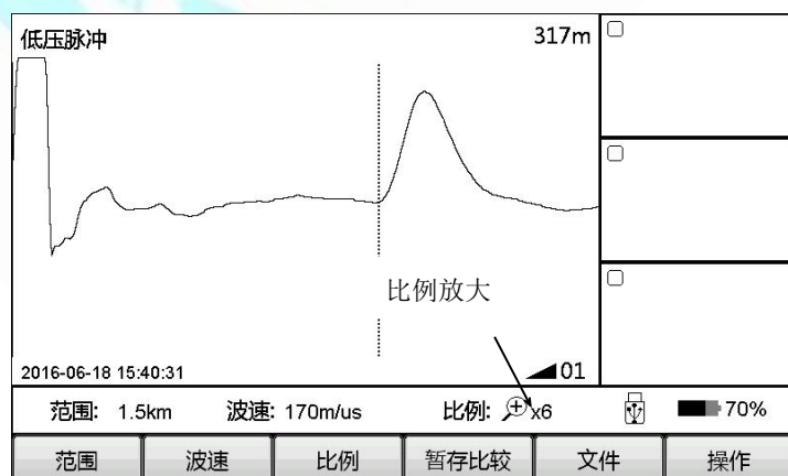
图 3-3-3 波形放大
