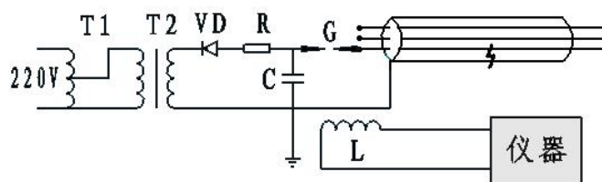
图 4-2-3 冲闪法原理图
