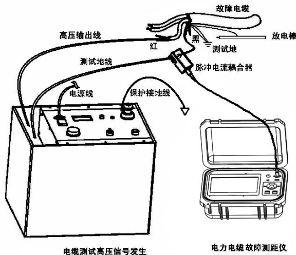
图 4-3-1 与电缆测试高压信号发生器配合使用
