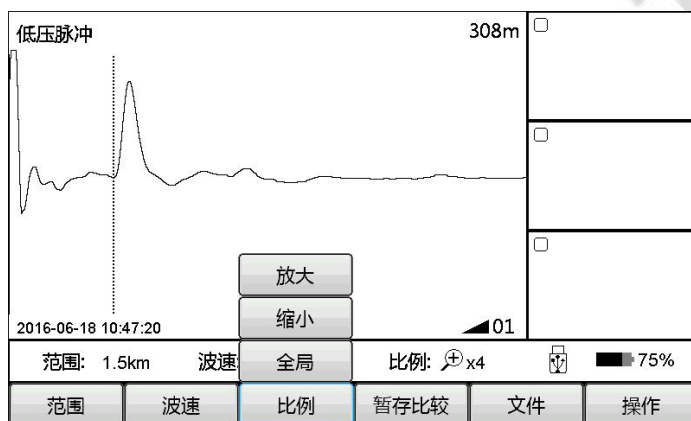
图 2-4-3
