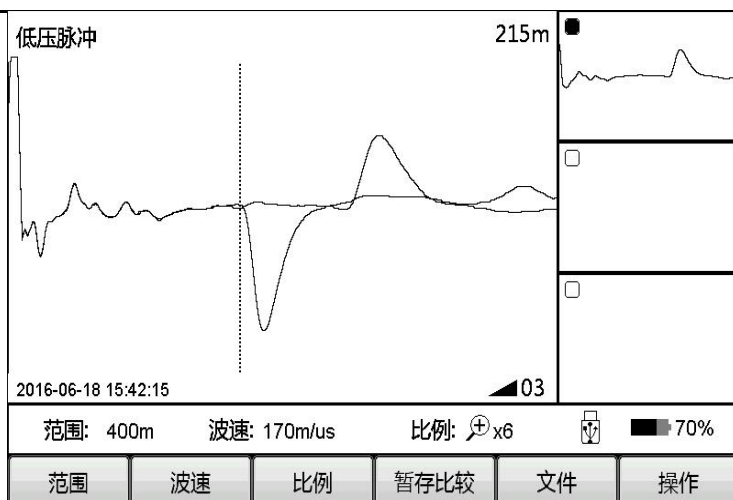
图 3-3-5 波形比较
