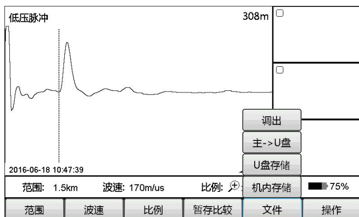
图 2-4-6
