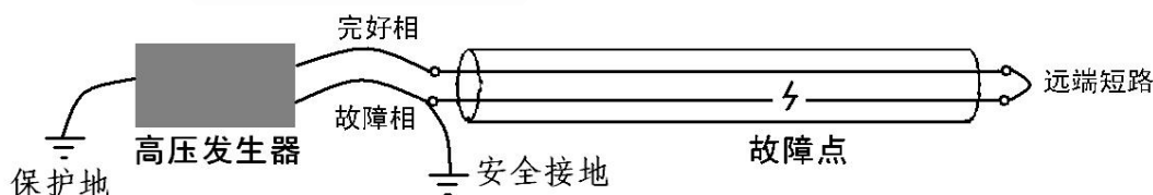
图 4-2-3 断线故障接线示意图
