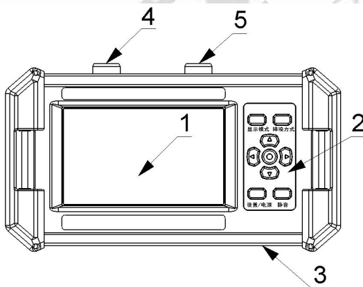
图 2-1-1 主机
