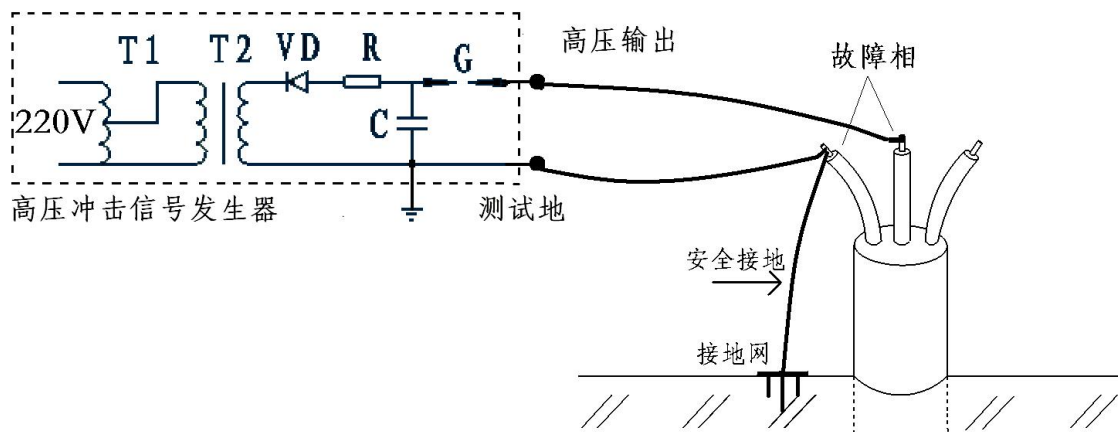
图 4-2-2 相间接法
