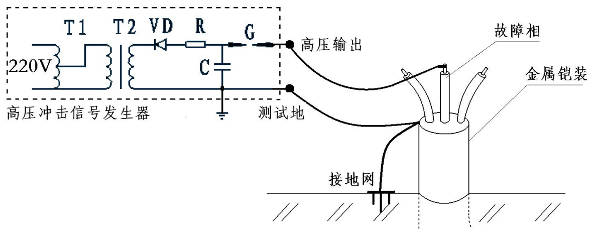
图 4-2-1 相对铠接法
