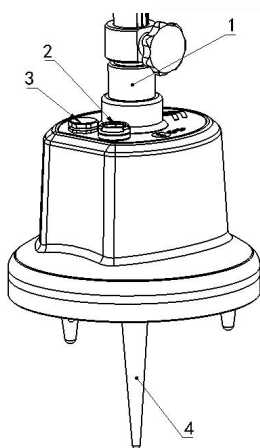
图 2-1-2 传感器
