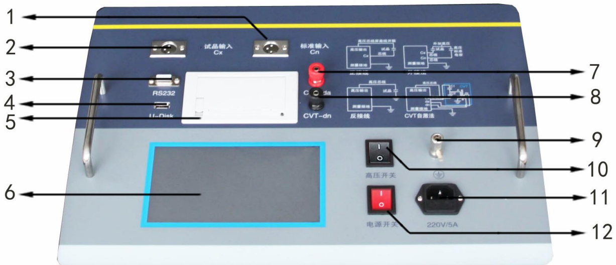
仪器面板 图三
