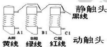
三断口信号线的连接
