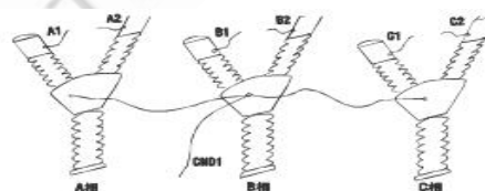
六断口信号线的连接
