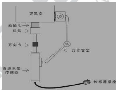
安装示意图
