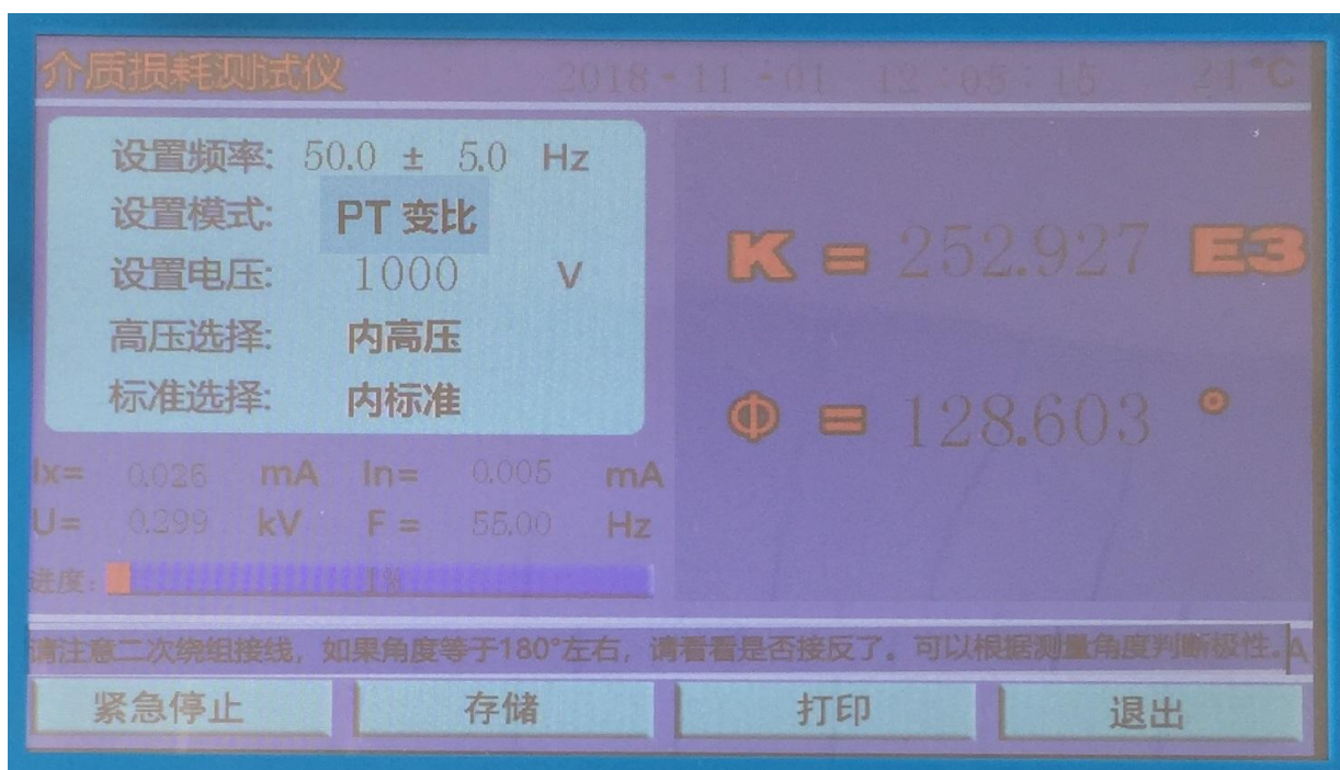
图十八 PT 变比测试结果
