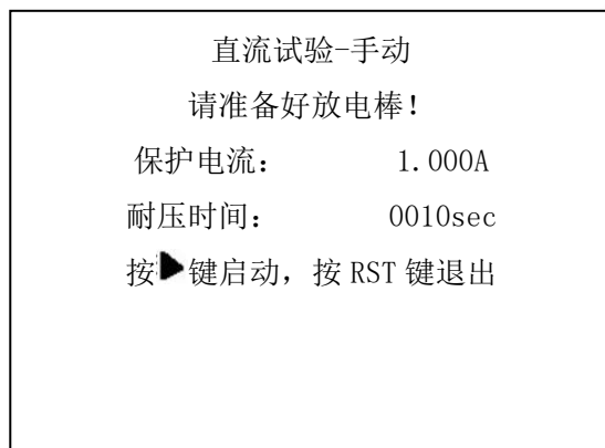
图 5-10 设置界面
