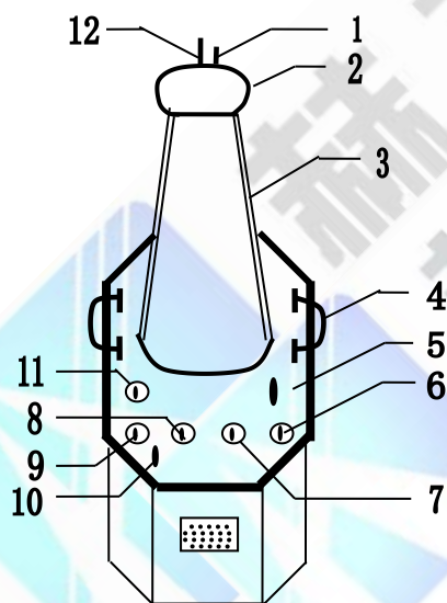
图 1：单台 YDJ-5KVA/50KV 工频耐压试验装置
