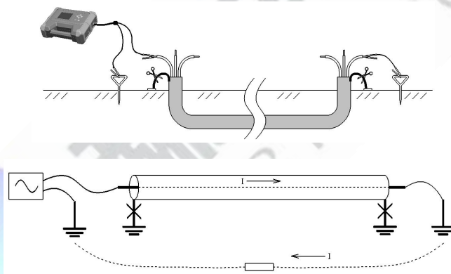
图 3-1-1 芯线—大地接线法
