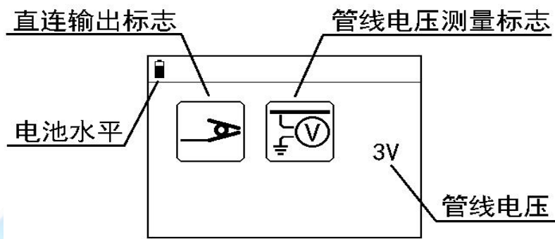
图 2-1-3 管线电压测量界面
