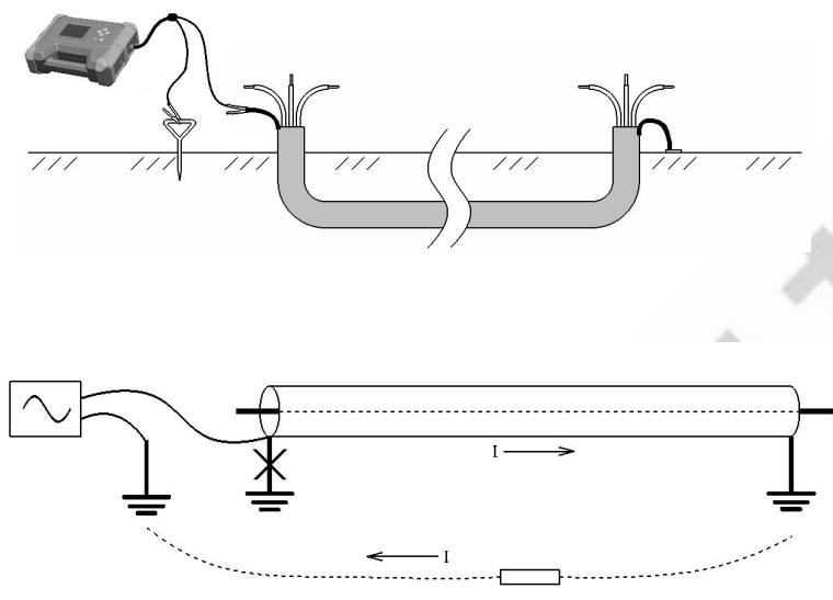
图 3-1-2 护层一大地接线法
