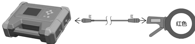
图 2-2-1 卡钳法附件连接
