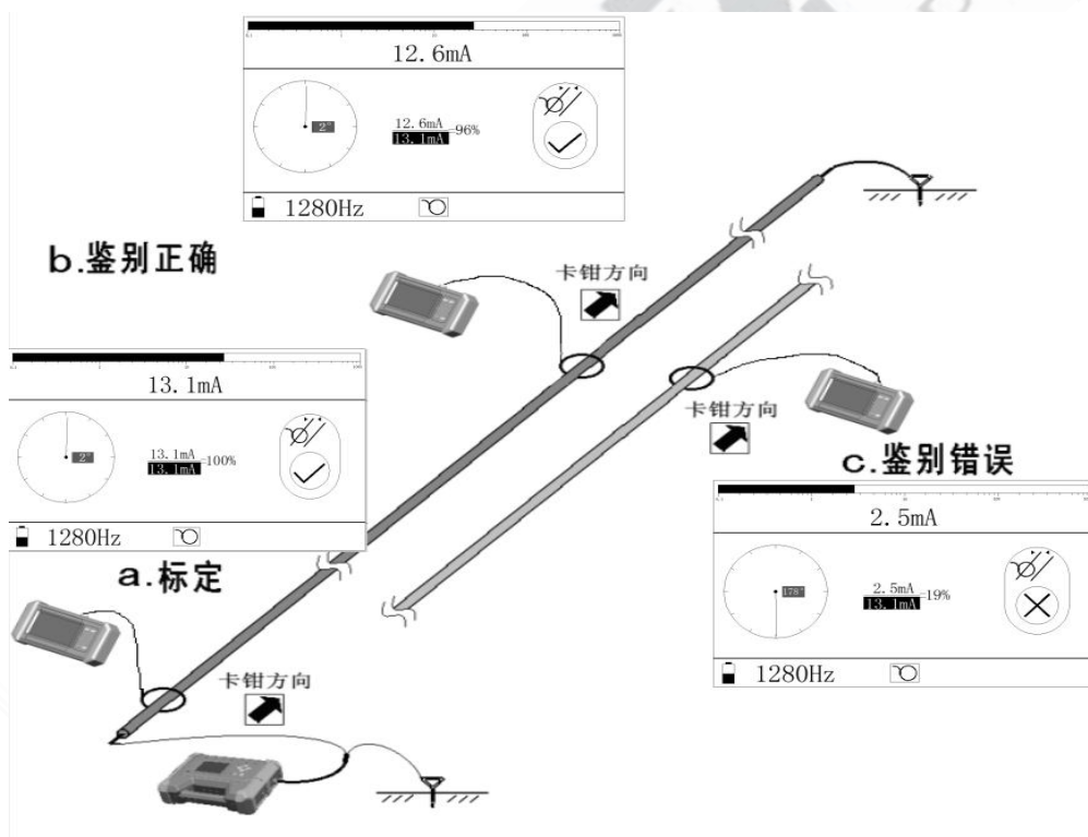
图 4-1-3 卡钳智能识别过程
