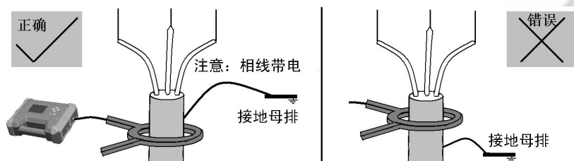
图 3-2-1 运行电缆卡钳耦合法 1（卡电缆本体）
