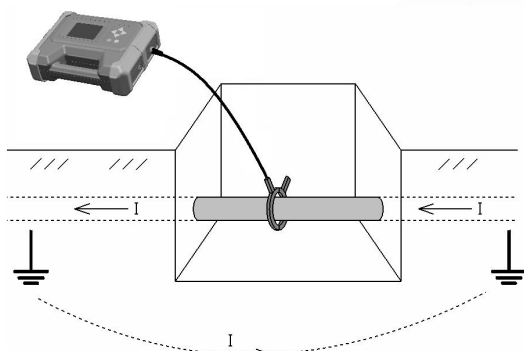
图 2-2-2 卡钳耦合法
