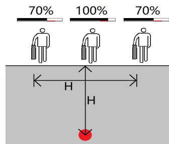
图 4-2-7 窄峰 70%法测深
