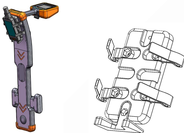
图 9-1-3 RTK 手持机安装背夹及安装效果
