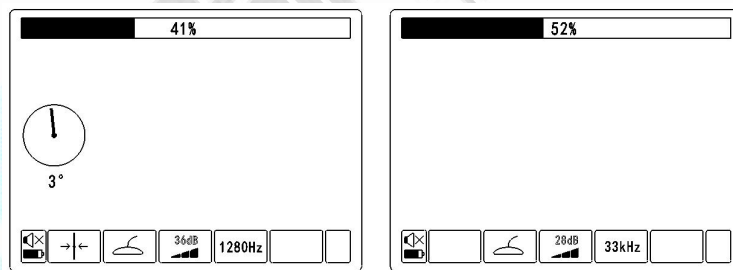
图 6-3-2 听诊器界面
