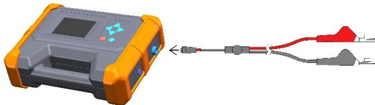
图 2-1-1 直连法附件连接
