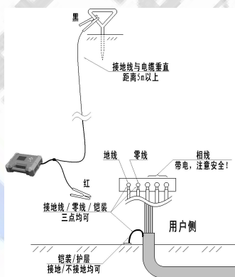
图 3-2-3 运行电缆零线 / 地线 / 护层注入法
