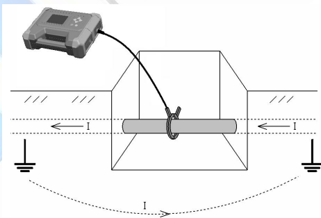
图 2-2-2 卡钳耦合法
