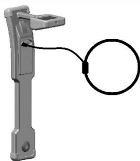
图 6-1-1 识别柔性卡钳连接
