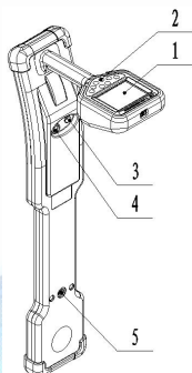
图 1-5-3 接收机 整体
