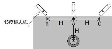
图 4-2-8 音谷 45° 法测深
