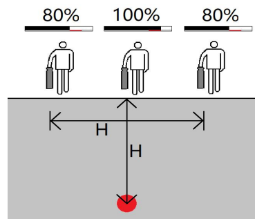
图 4-2-6 宽峰 80%法测深
