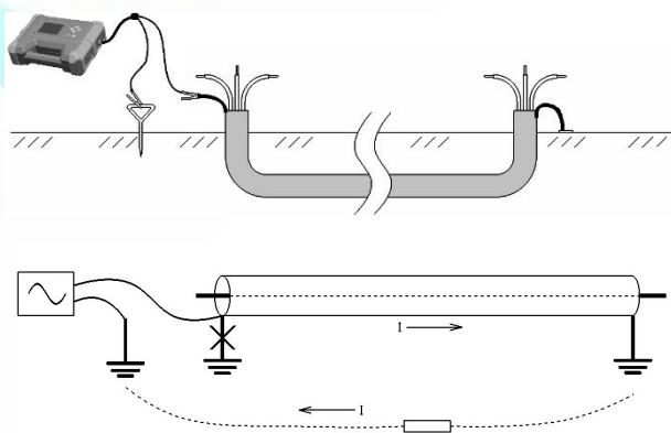
图 3-1-2 护层一大地接线法
