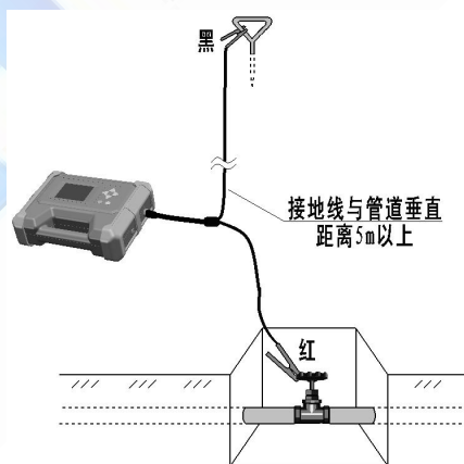
图 2-1-2 直连法接线
