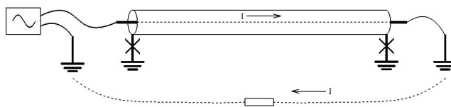
图 3-1-1 芯线一大地接线法
