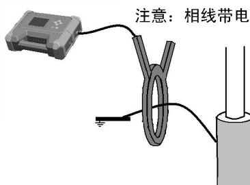
图 3-2-2 运行电缆卡钳耦合法 2（卡电缆接地线）
