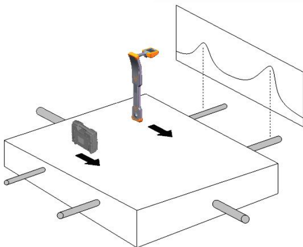
图 4-1-8 辐射法区域探查
