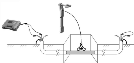
图 6-3-3 听诊器识别
