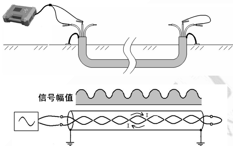
图 3-1-5 相间接法
