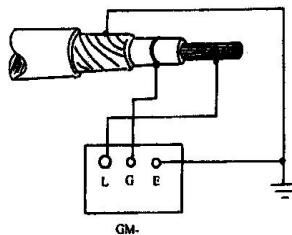
屏蔽电缆绝缘测试接线图
