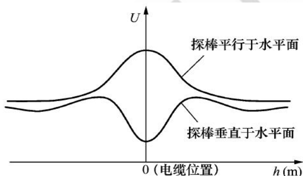
路径探测接收幅值与位置关系图
