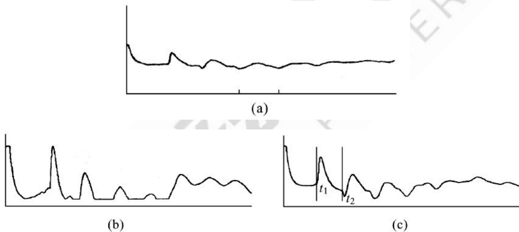
(a) 冲击电压为 15kV 实测波形；(b) 增大输出幅度
