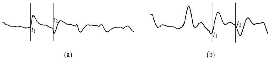
(a) 冲击电压为 8kV 实测波形；(b) 冲击电压为 15kV 实测波形
