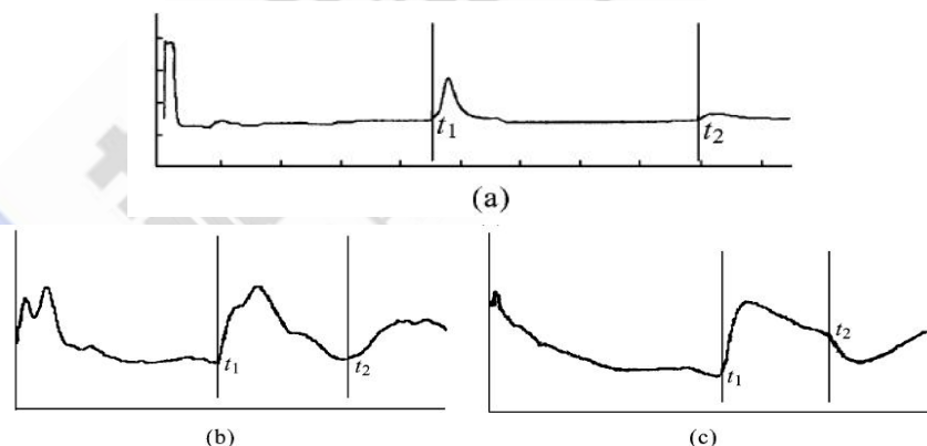
(a) 脉冲法实测波形；(b) 冲闪电流冲击电压为 21kV 实测波形； (c) 冲闪电压法冲击电压为 21kV 实测波形
