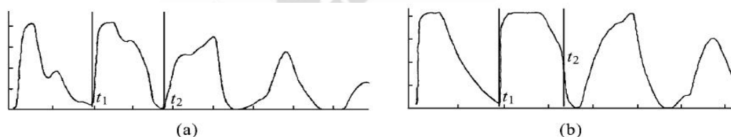
(a) 电流法冲击电压为 12kV 实测波形；(b) 电压法冲击电压为 12kV 实测波形；
