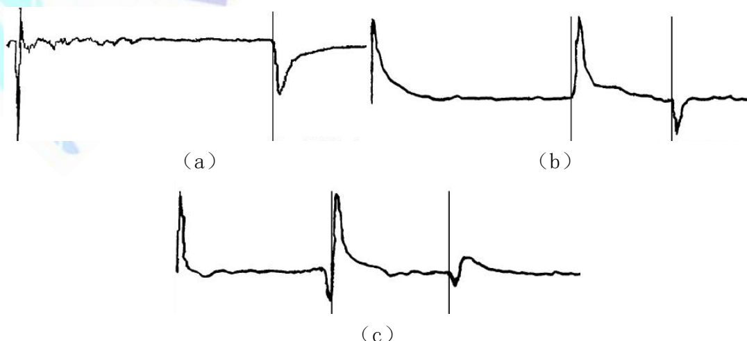
图 26 北海供电局电力电缆实测波形
