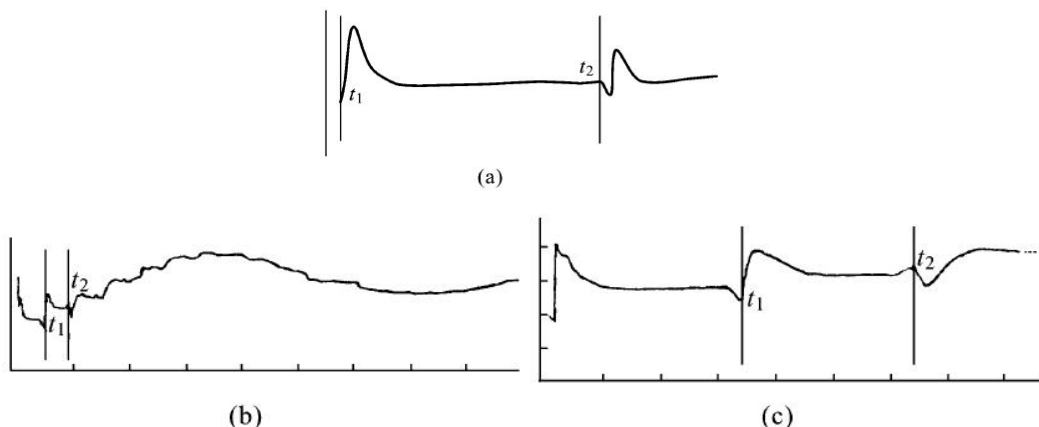
(a) 脉冲法实测波形；(b) 冲击电压为 5kV 实测波形；(C) 冲击电压为 5kV 实测扩展波形
