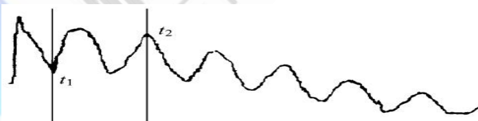
图 12 西宁供电局电力电缆实测波形
