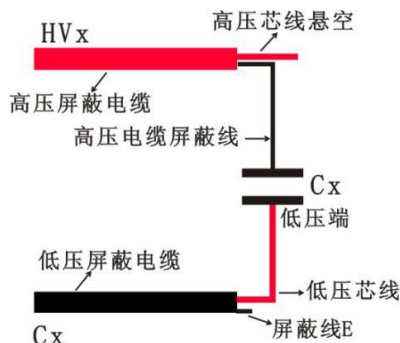
图 6 反接法
