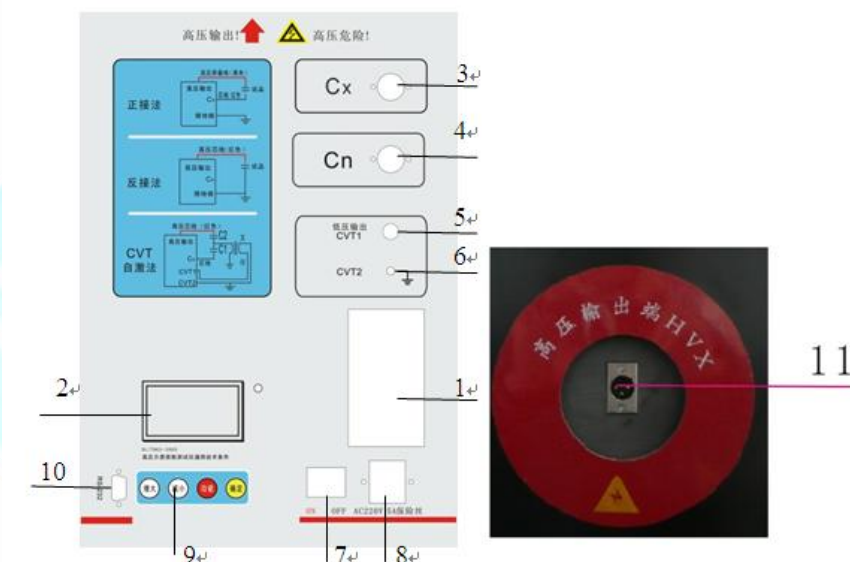
图 1 仪器面板和侧面
