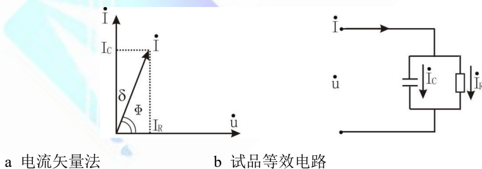
图 4 试品等效电路
