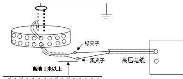
图 19 标准电容器 BR26、介损器 DB-100 等反接线（接地试品）接线法
