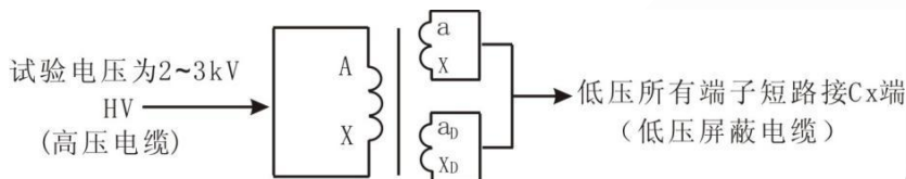
图 12 常规接线法
