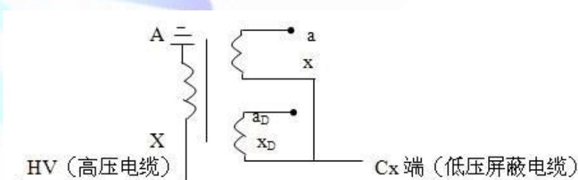
图 14 末端加压法接线
