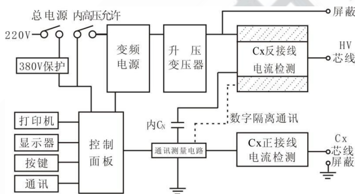
图 2 仪器原理图
