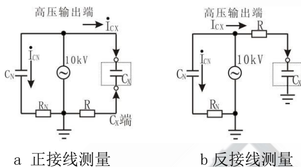
图 3 测量原理图
