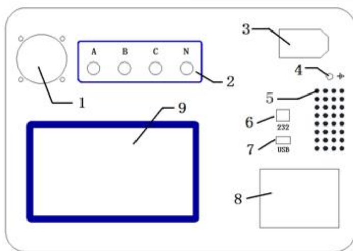
图 5.1 面板图
