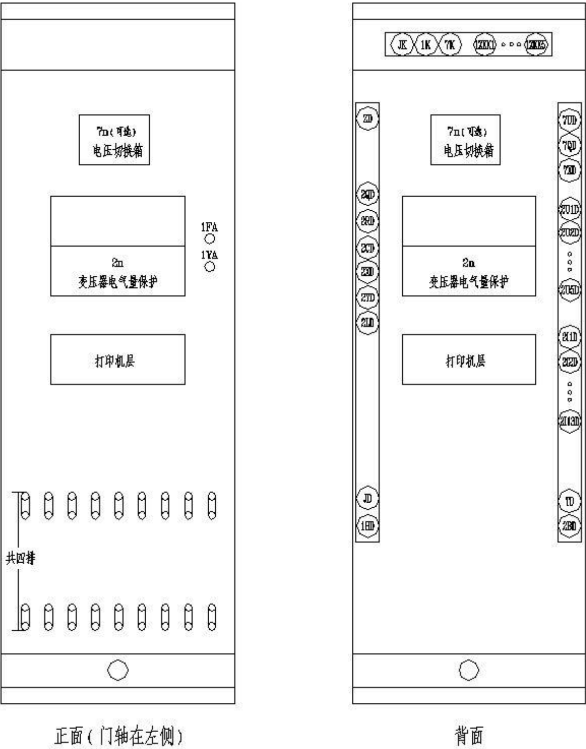
图A.5 变压器保护屏A (屏B) 屏面布置示意图 (有发电机出口断路器“五屏”方案)
