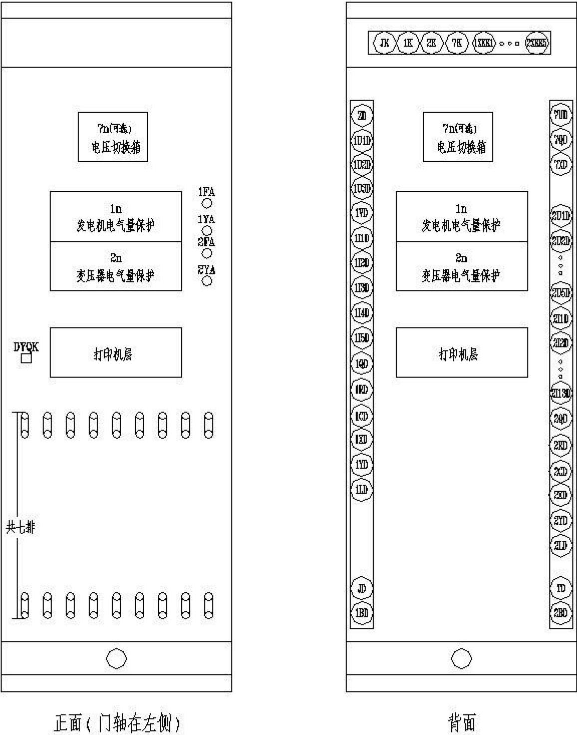
图A.7 发变组保护屏A (屏B) 屏面布置示意图 (有发电机出口断路器“三屏”方案)
