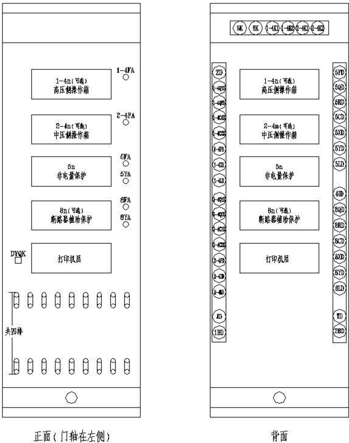
图 A.2 发变组保护屏 C 屏面布置示意图（无发电机出口断路器方案）
