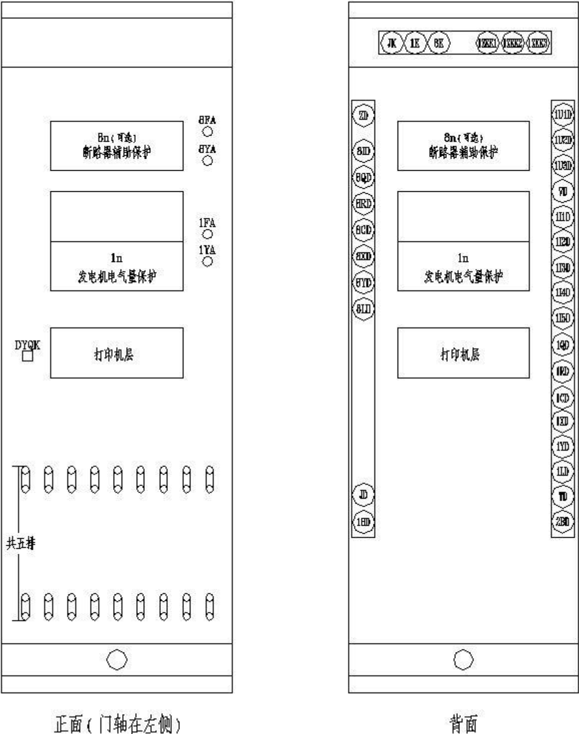
图 A.4 发电机保护屏 B 屏面布置示意图 (有发电机出口断路器“五屏”方案)
