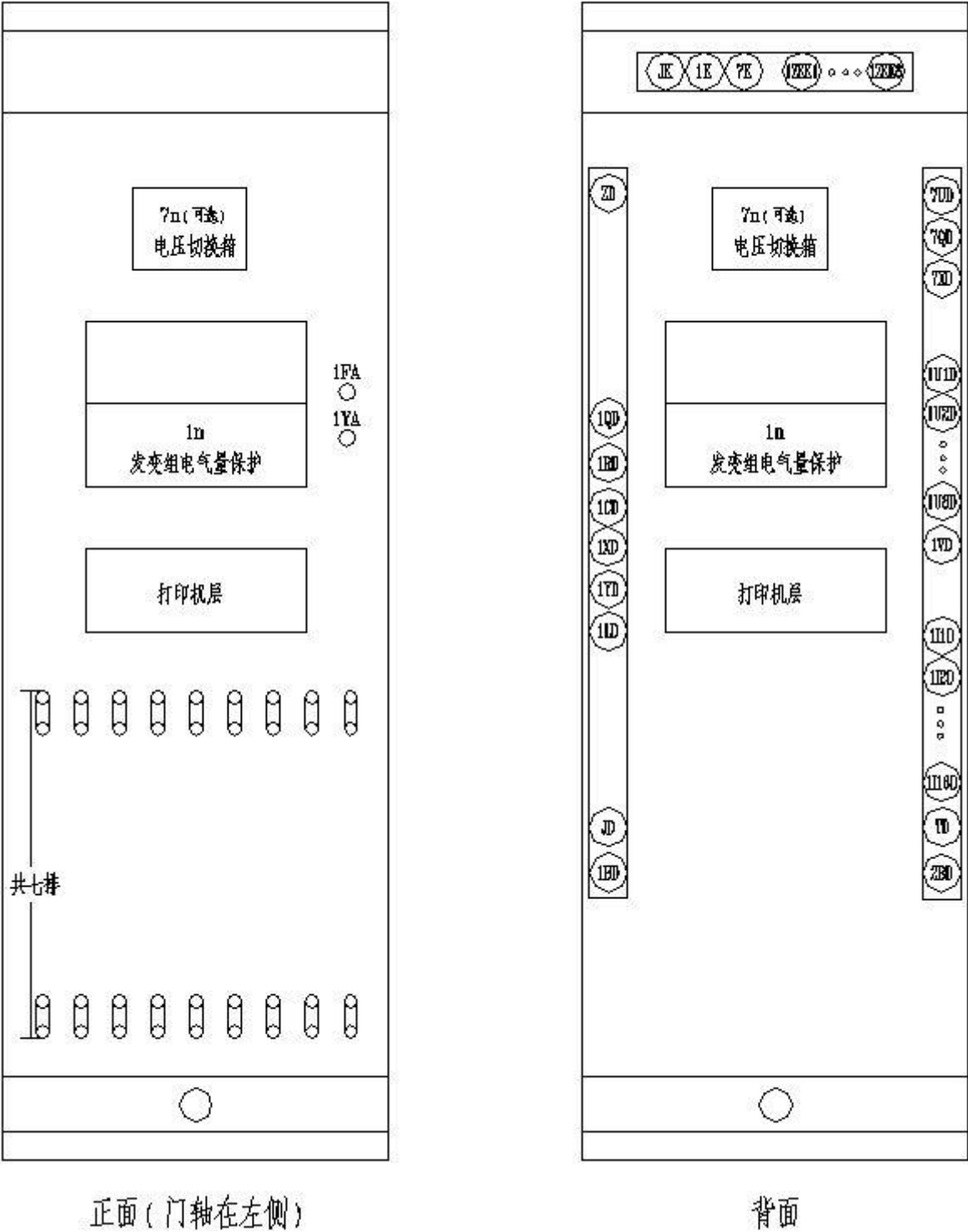
图 A.1 发变组保护屏 A (屏 B) 屏面布置示意图 (无发电机出口断路器方案)
