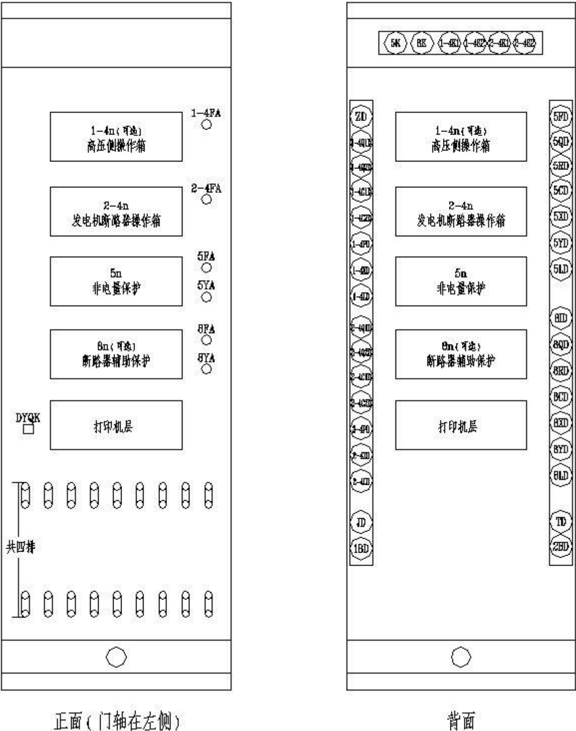
图 A.8 发变组保护屏 C 屏面布置示意图（有发电机出口断路器“三屏”方案）
