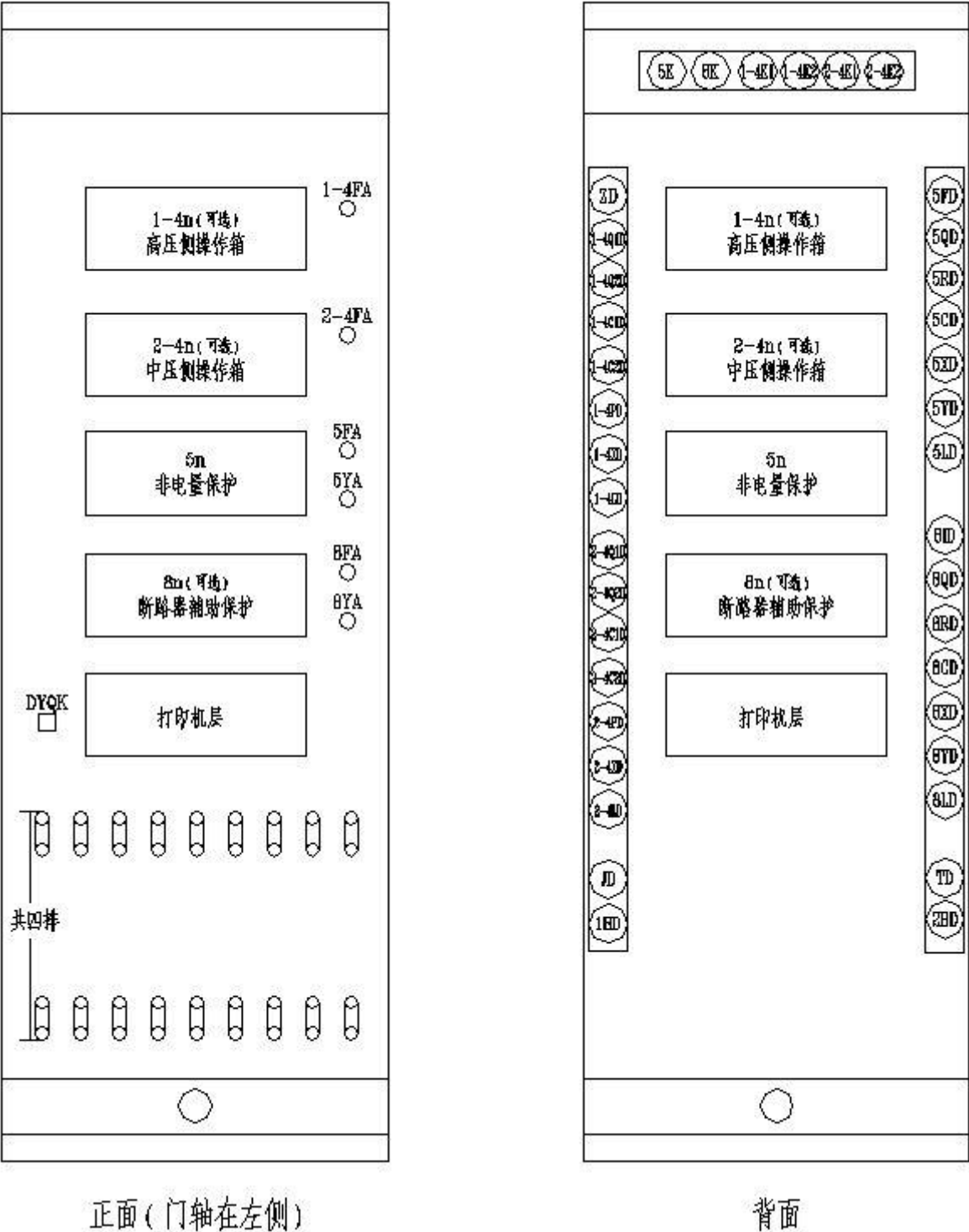
图 A.6 发变组保护屏 C 屏面布置示意图 (有发电机出口断路器“五屏”方案)
